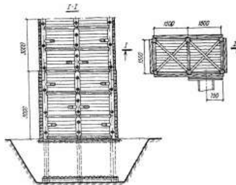
Рис. 9. Двухсекционный деревянный водобросной колодец высотой до 6 м
