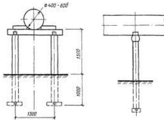
Рис. 2. Двухстоечная закопная опора высотой 1,5 м
