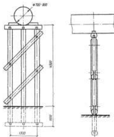
Рис. 3. Трехстоечная закопная опора высотой 4 м
