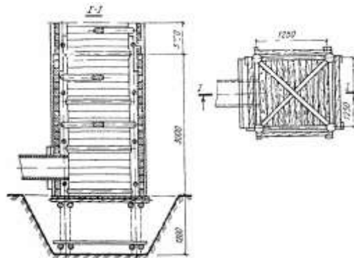
Рис. 7. Односекционный деревянный водосбросной колодец высотой до 6 м
